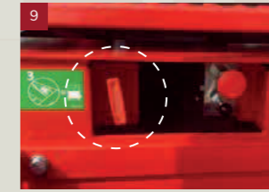
Manuel İndirme Valfi: İşletim sistemi başarısız olduğunda veya pil gücü platformun inişine izin vermeyecek kadar düşük olduğunda, makineyi indirmek için bu valfi kullanabiliriz.
